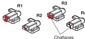
Contrapienza N.º de identificación del chaflán 1/2 N.º de identificación del chaflán 3/4
